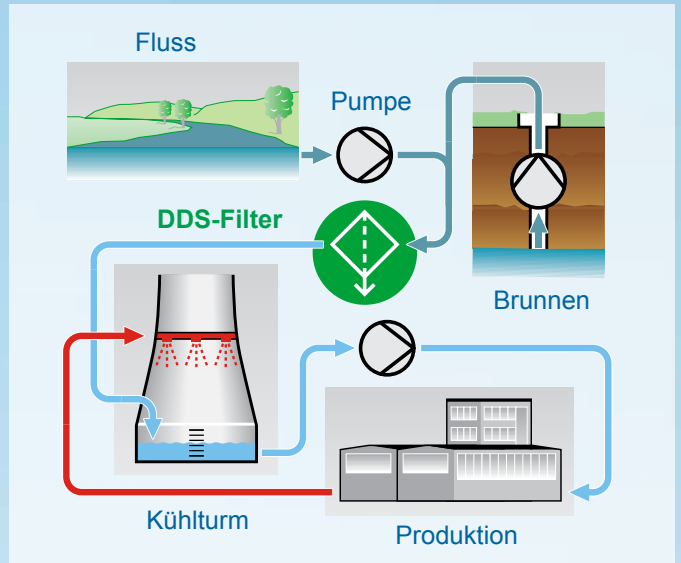
Filtration von Zusatzwasser
