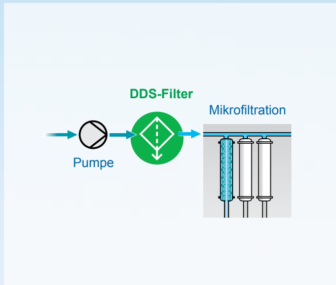
Vorfiltration
