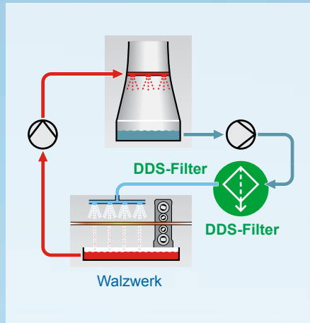
Schutz von Spitzdüsen
