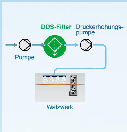
Schutz der Druckerhöhungspumpe
