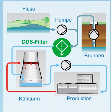
Filtration von Zusatzwasser
