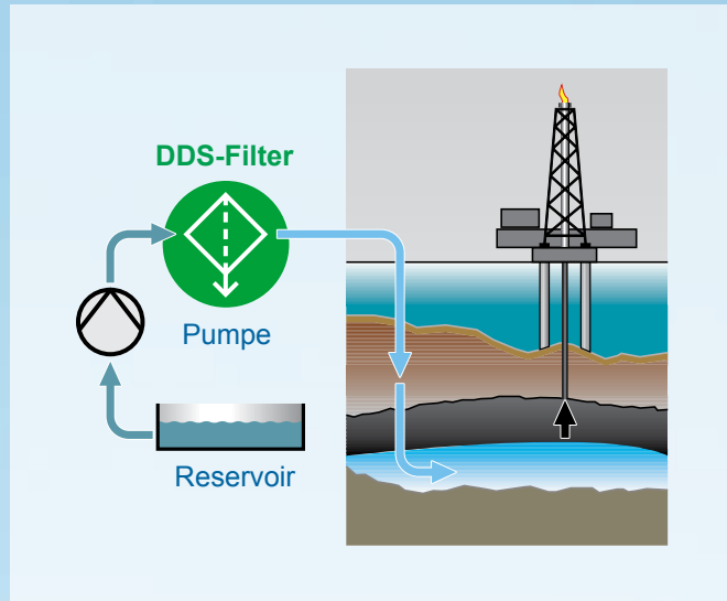
Filter für Offshore-Technik
