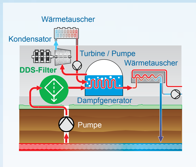
Filter für Thermalwasser
