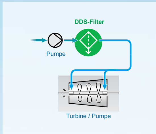
Filtration von Sperrwasser
