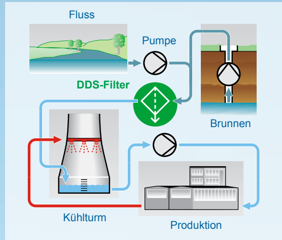
Filtration von Zusatzwasser
