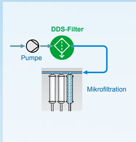
Vorfiltration
