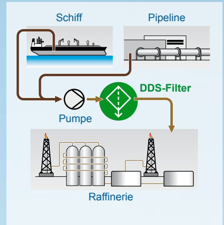
Rohöl-Filtration
