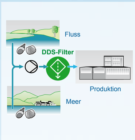
Muschelfiltration
